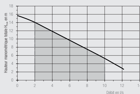
Courbe caractéristique de pompe
