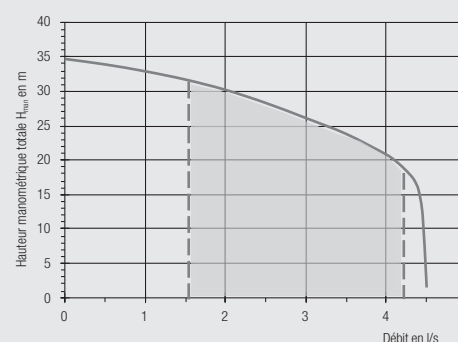
Courbe caractéristique de pompe
